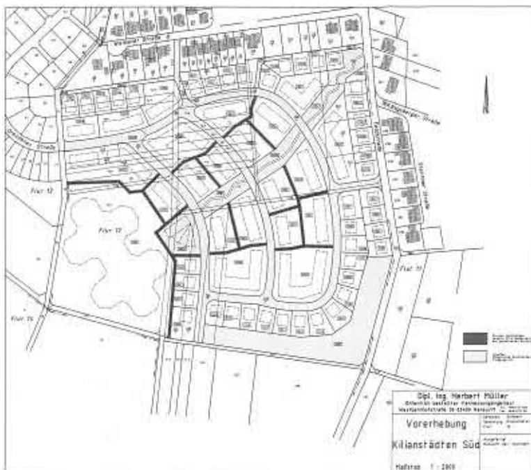
Abbildung 31: Entwurf Umlegungsplan Dipl. Ing. Herbert Müller
